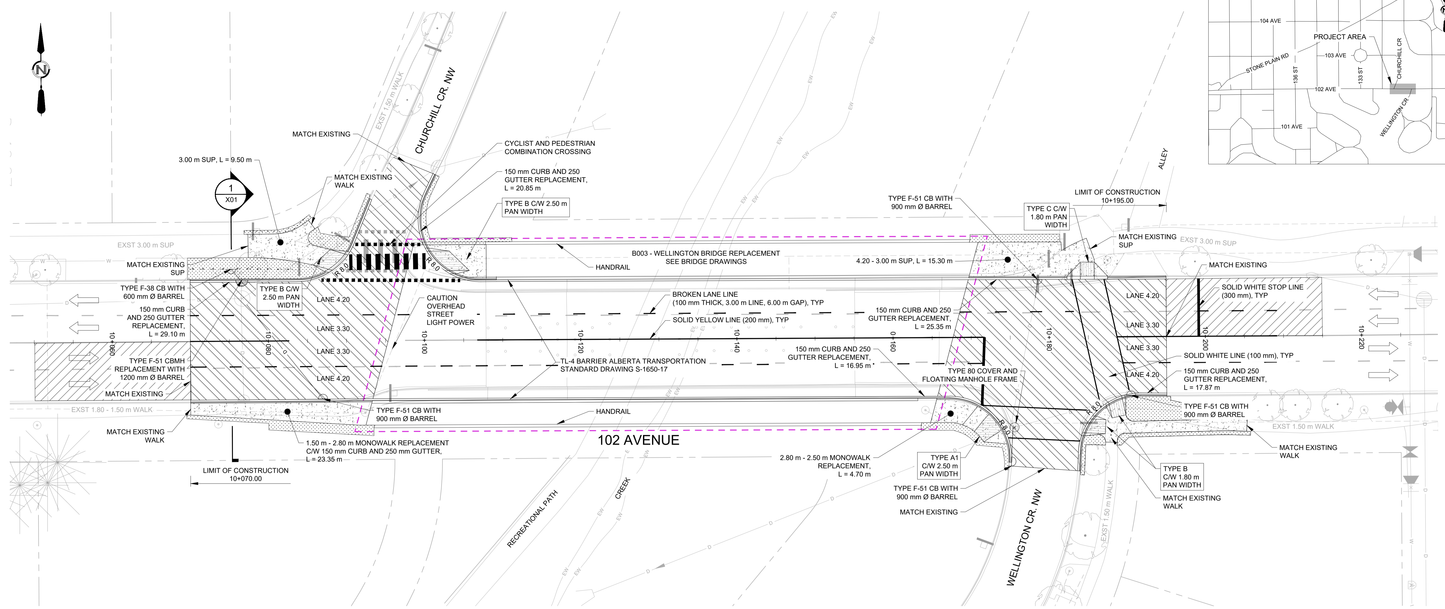
1 PLAN 1:250 102 AVENUE
