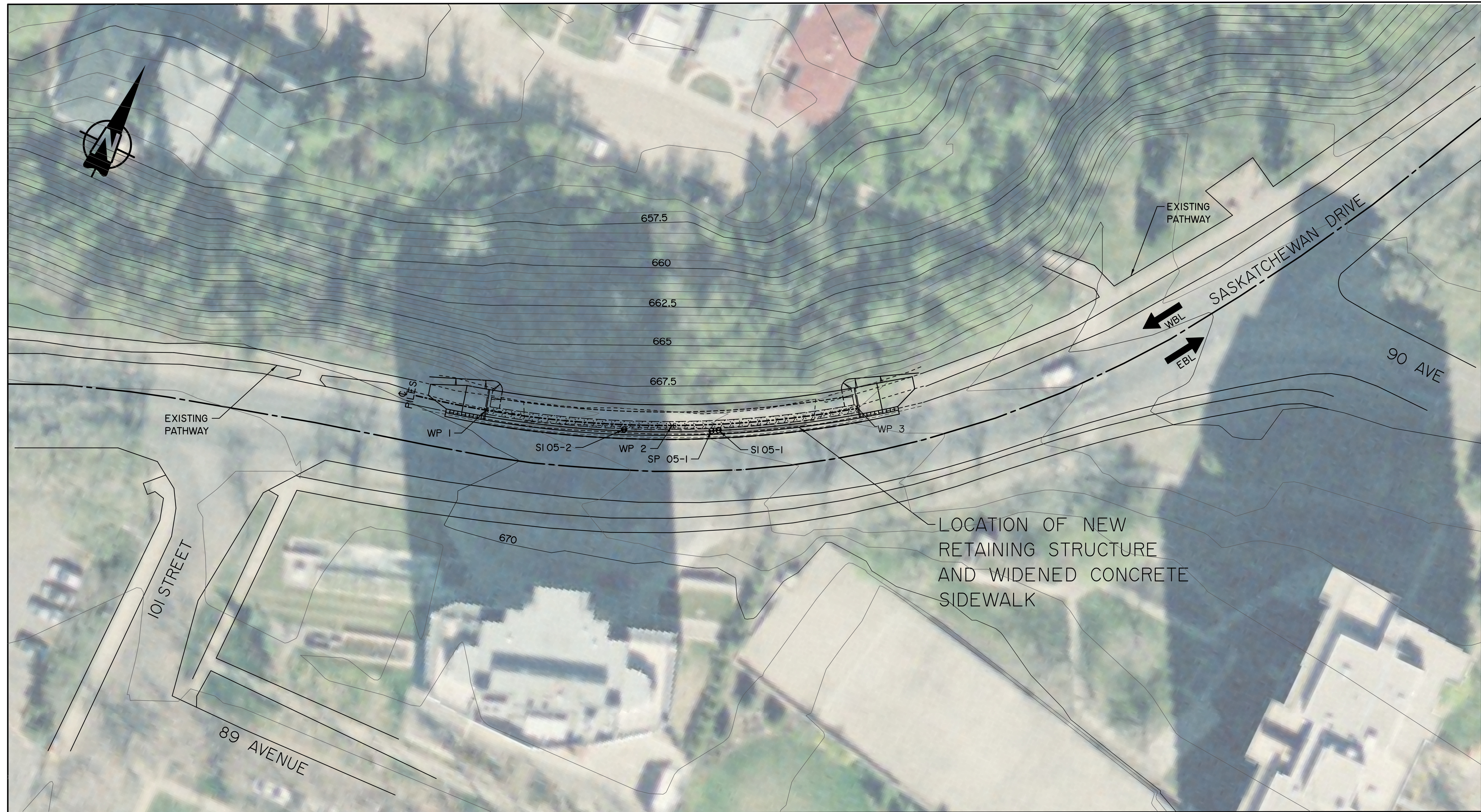
SITE MAP 1:300
